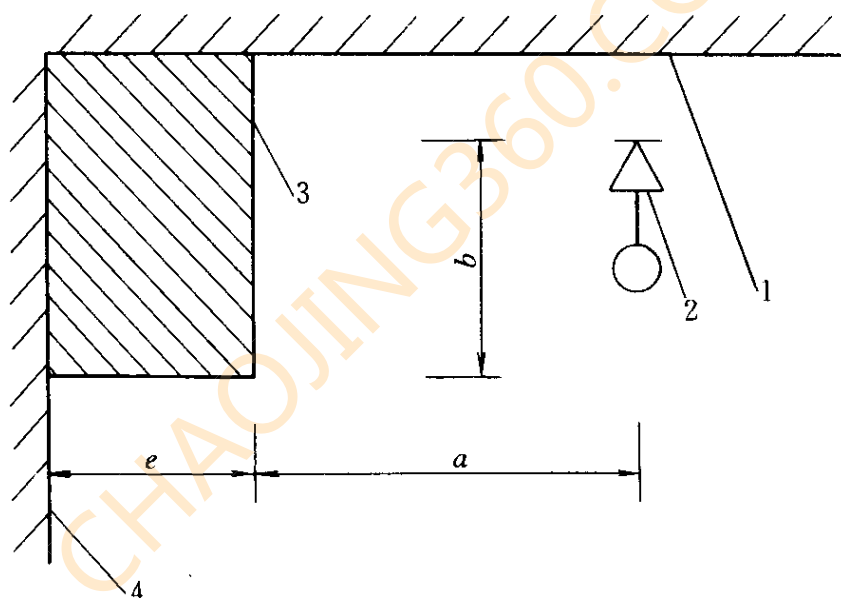
图 7.2.5 喷头与靠墙障碍物的距离
