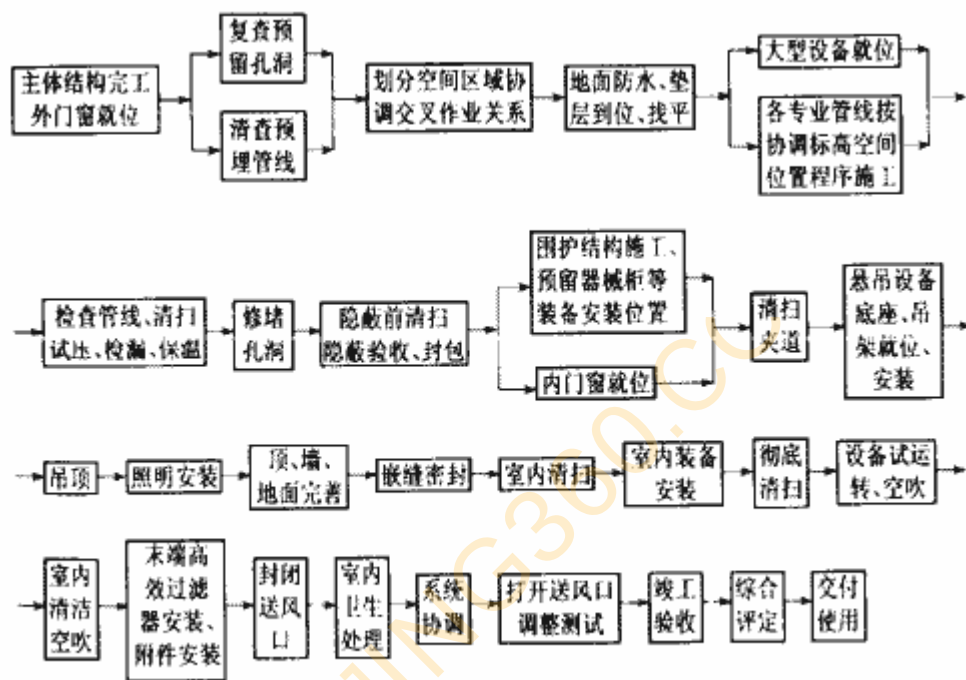
图 10.1.2 洁净手术室施工程序
