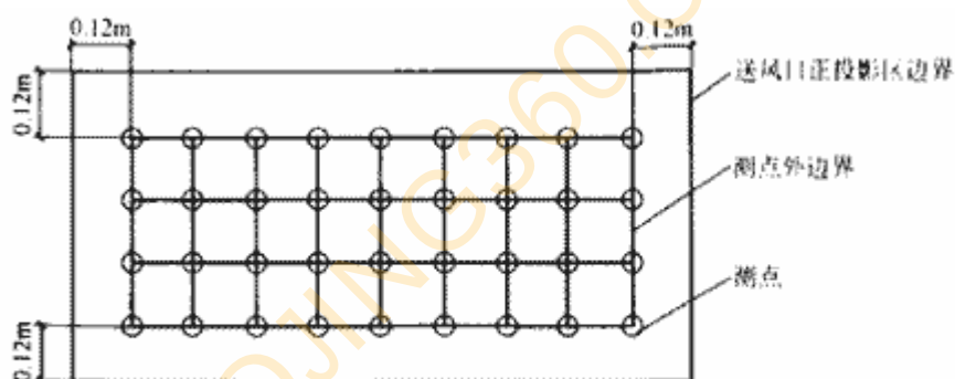
图 10.3.5 截面风速测点平面布置
