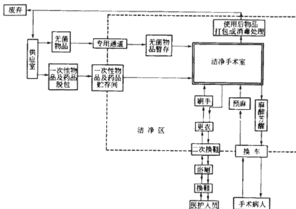
图 5.2.5 洁净手术部人、物净化流程
