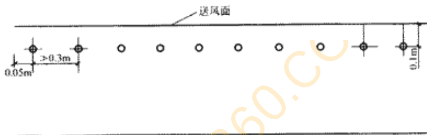
图 10.3.6 送风面速度测点断面布置
