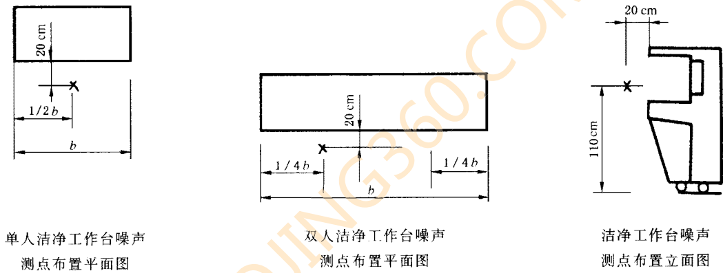
图 8 洁净工作台噪声测点布置图
