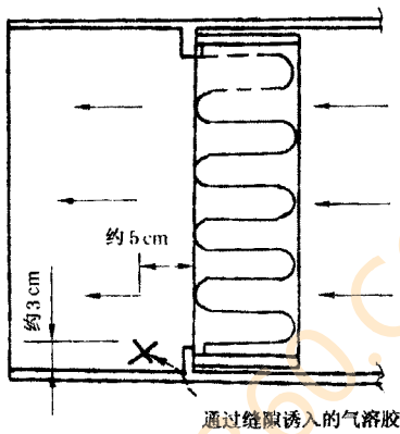
图 3 气溶胶通过水平层流洁净工作台缝隙诱入测点位置的示意图
