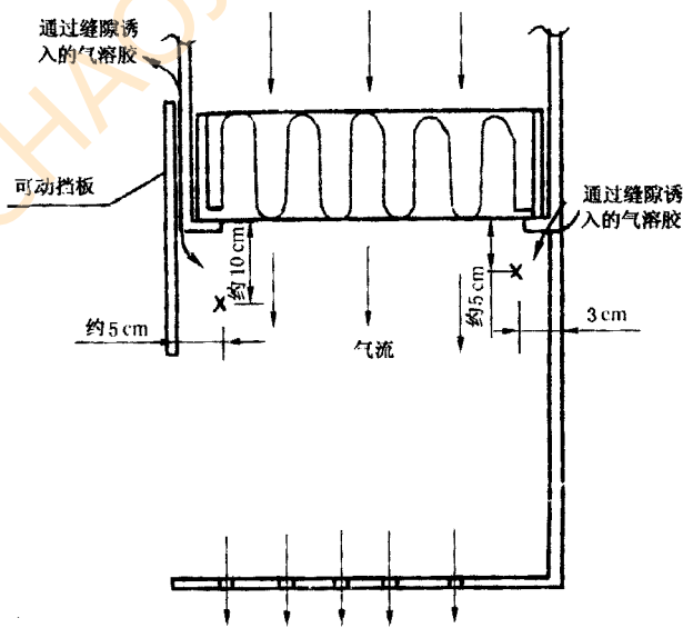
图 4 气溶胶通过垂直层流洁净工作台缝隙诱入测点位置的示意图
