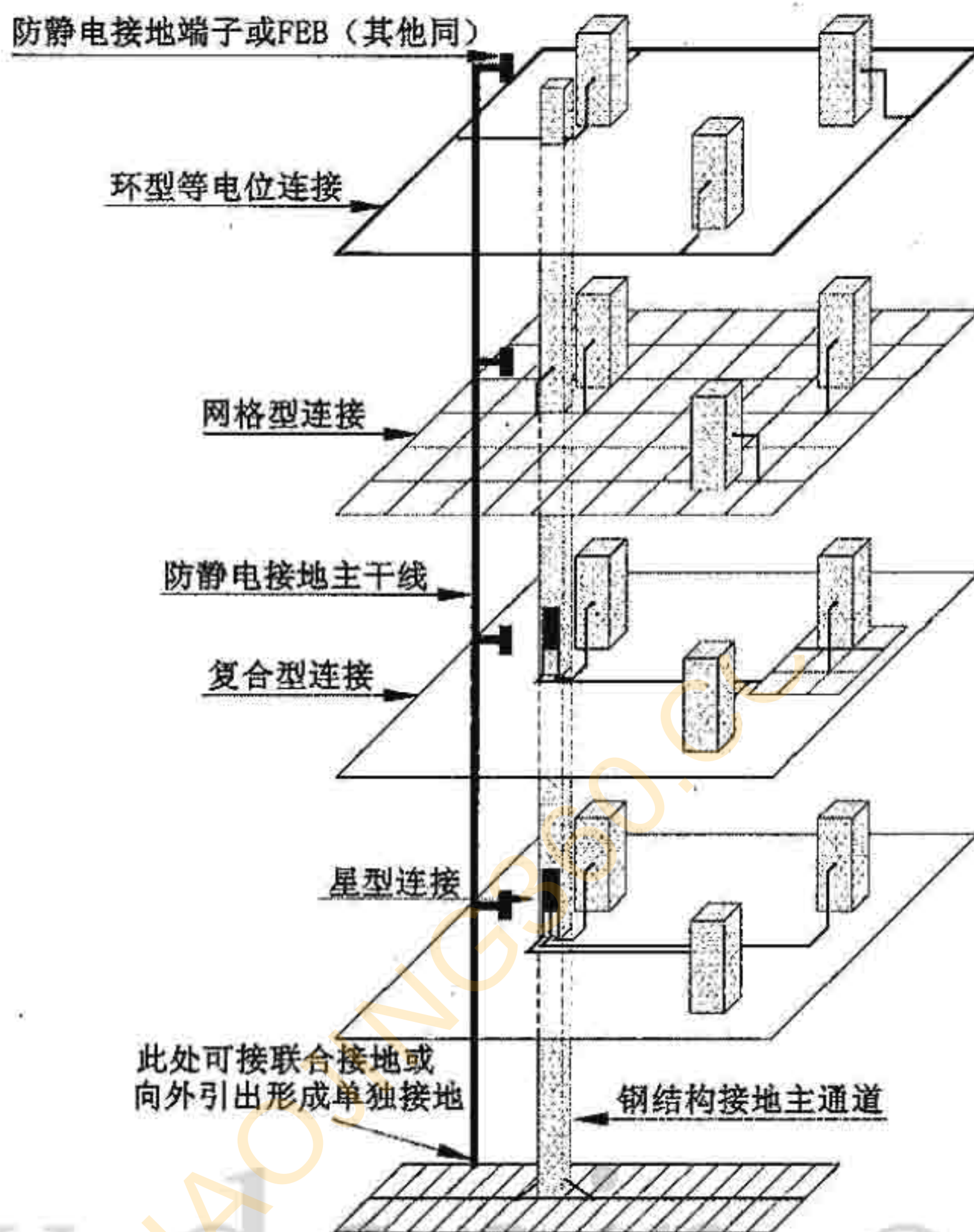
图2 防静电接地系统典型布置
