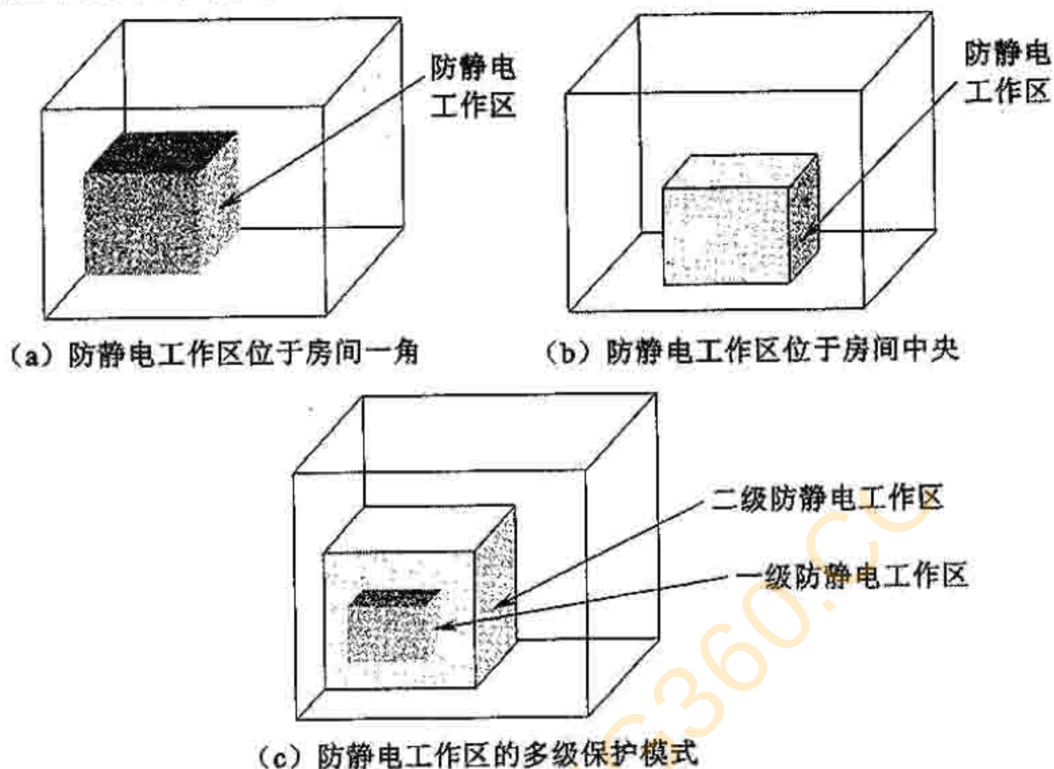
图 1 防静电工作区边界的空间界定
